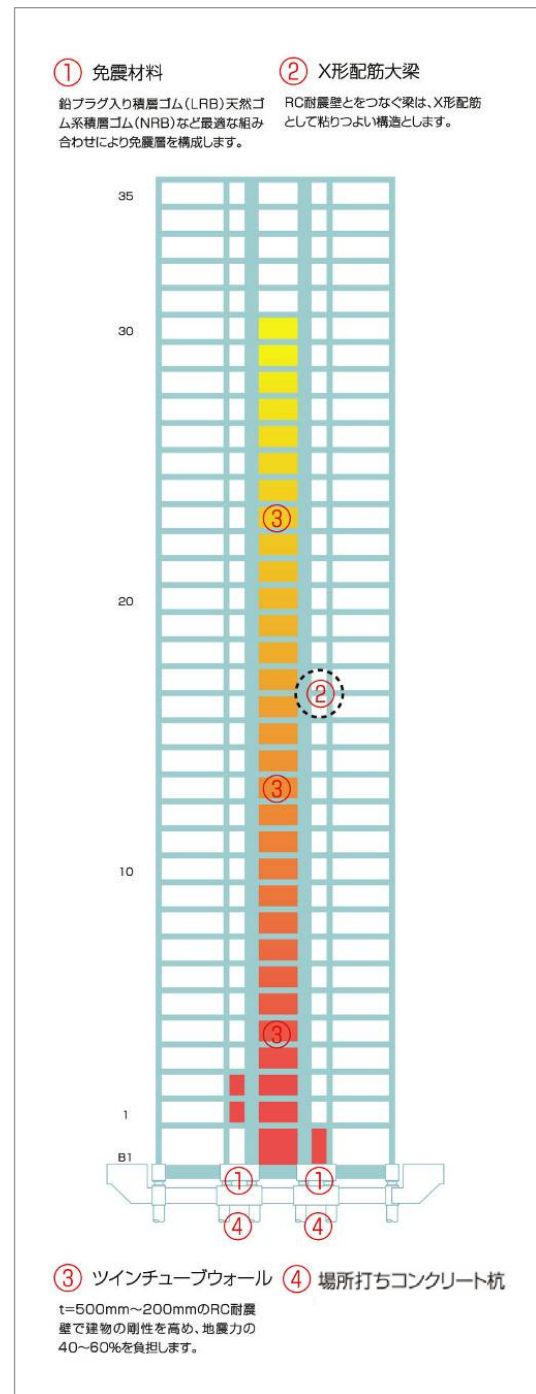
免震性能概念図
