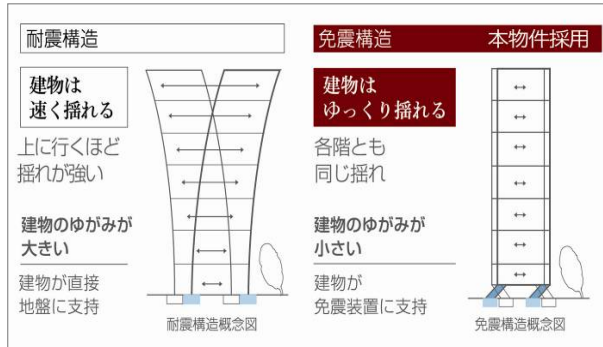
一般的な耐震構造と免震構造
